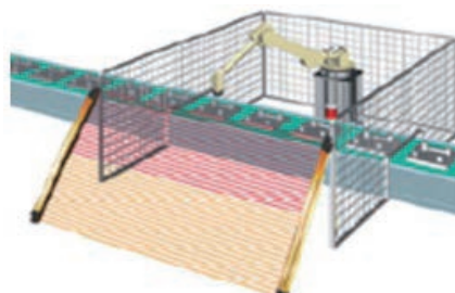
警告区与停机区
